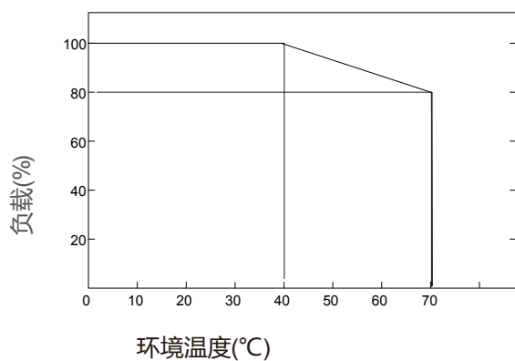
■ 减额曲线
