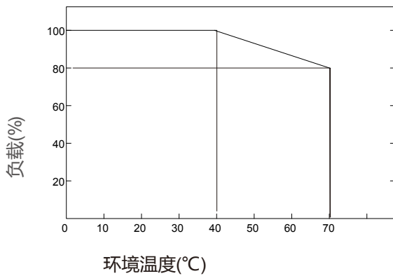
■ 减额曲线
